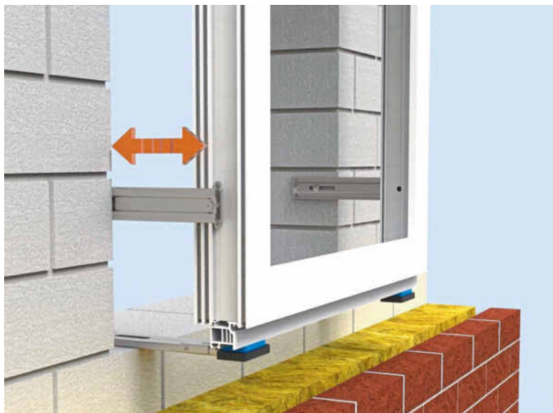
Ausgereift und mit abZ: Vorwandmontagesystem JB-D Plus von SFS
