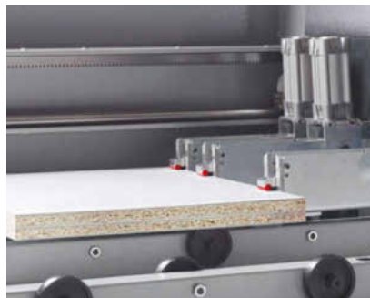
Sicheres Klemmen von Plattenpaketen und einzelnen, kleinen Plattenmaterialien
