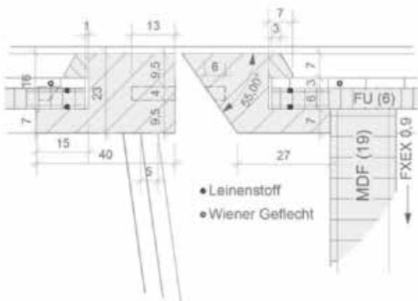
Horizontalschnitte: Detailausbildung des seitlichen Türanschlags
