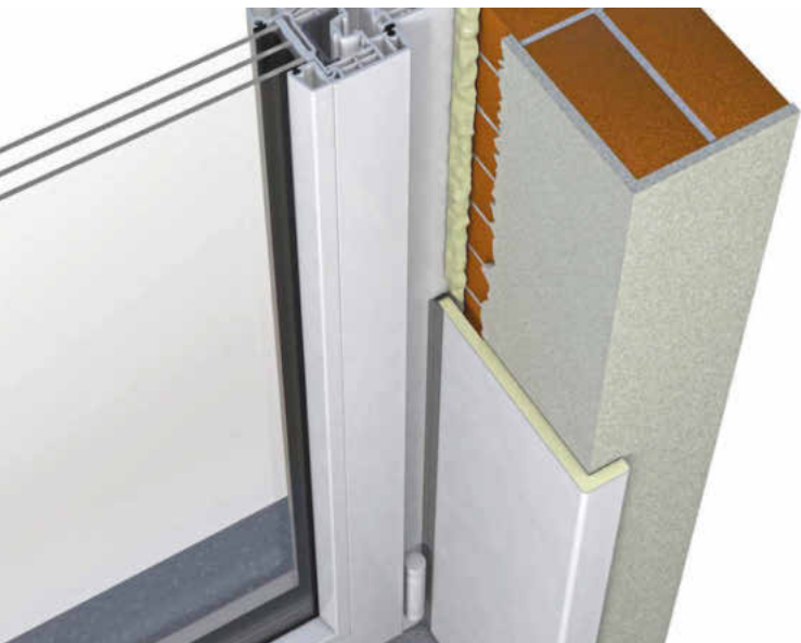
Reno-Therm-Winkelleisten mit Haftbeschichtung in Putzstruktur von Beck+Heun
